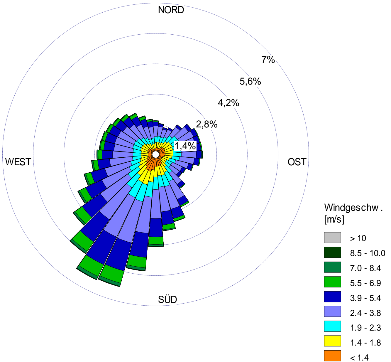
Abbildung 2: Windrichtungsverteilung und Standortdaten der Station Lingen. Zeitraum: 1997 bis 2006
